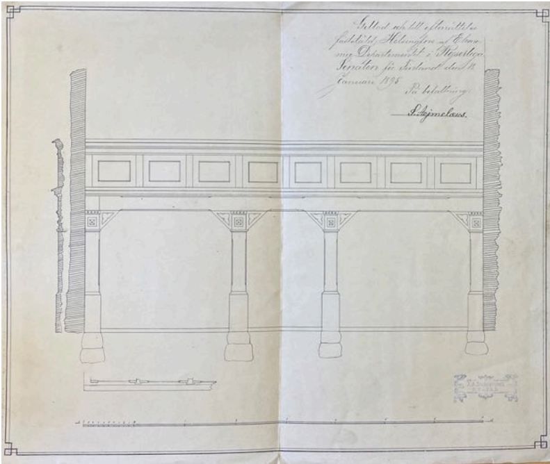
Zachariassenin Houtskarın kirkon urkuparven hyväksytyt piirustukset. Zachariassens godkända ritning till orgelläktare i Houtskärs kyrka.
